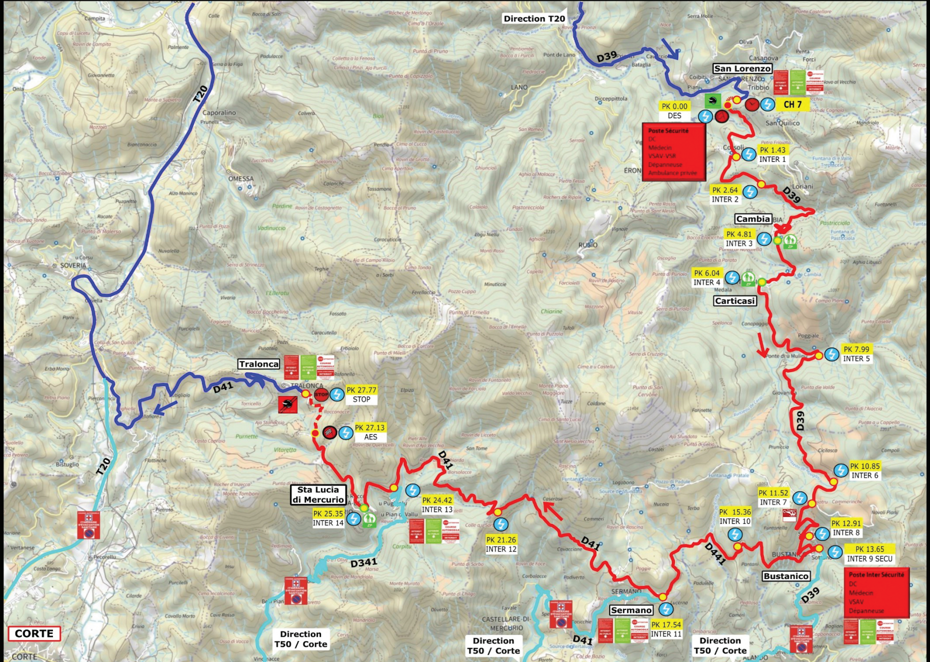
ES7: San Lorenzo - Tralonca - 27.13 Km
